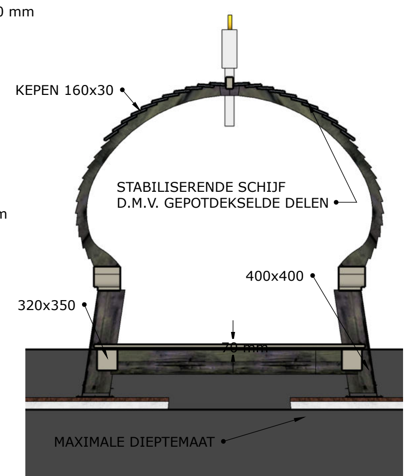
DWARSDOORSNEDE
