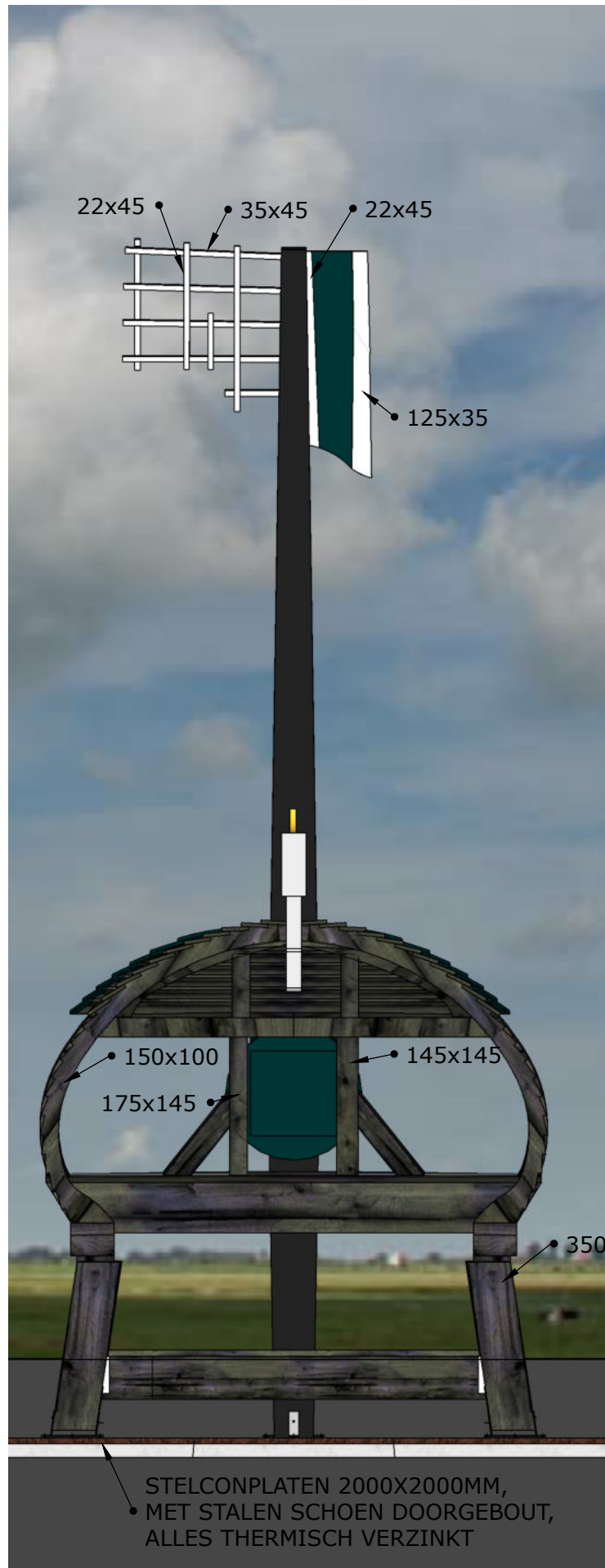
ACHTERAANZICHT
