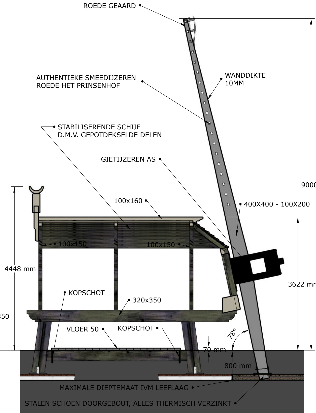
LANGSDOORSNEDE
