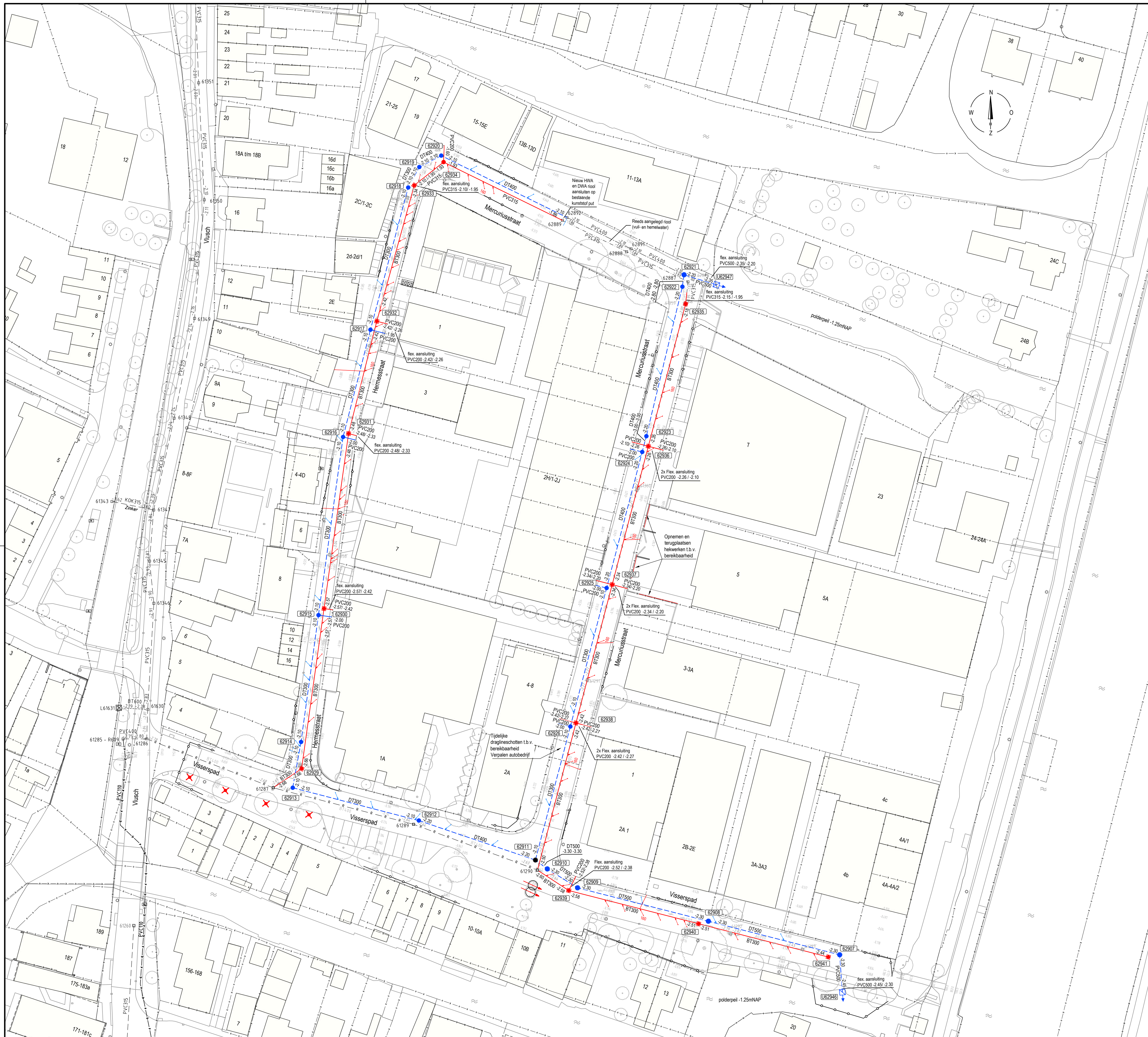
Situatieoverzicht Schaal 1:500
