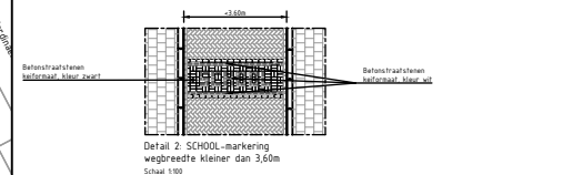
Detail 2: SCHOOl-markering wegbreedte kleiner dan 3,50m Schaal 1:50
