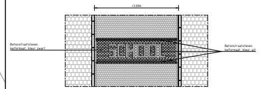
Detail 1: SCHOOl-markering wegbreedte groter dan 3,50m Schaal 1:50
